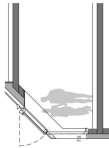
SCHNITT A
