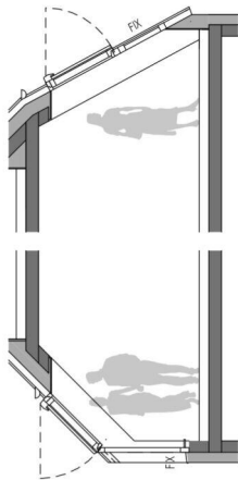
SCHNITT A
