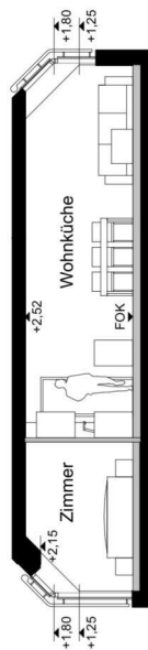
Querschnitt M:1:150 Wohnküche und Zimmer
