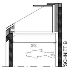
SCHNITT B3
