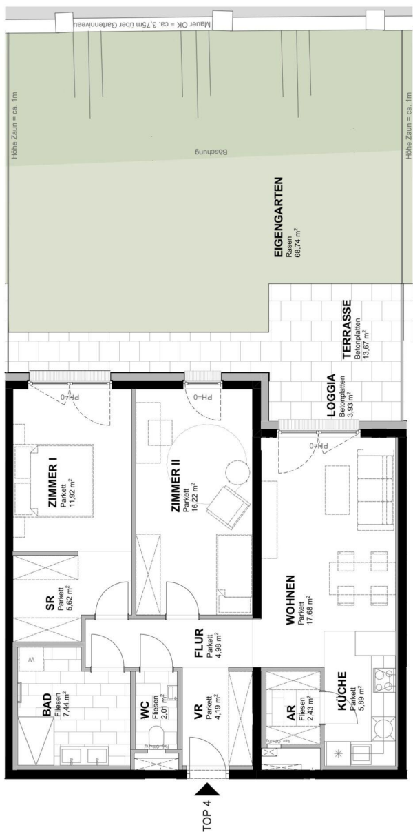
Übersichtsplan Erdgeschoss
