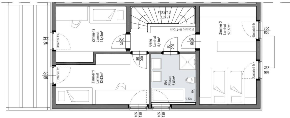
OBERGESCHOSS
