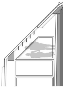
SCHNITT C
