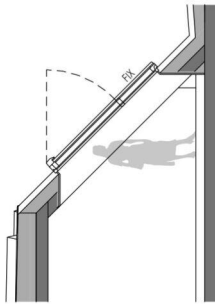
SCHNITT B
