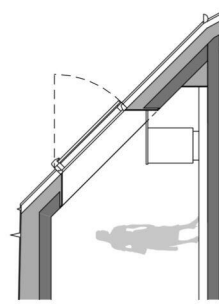
SCHNITT E
