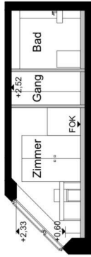
Querschnitt M:1:150
