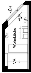
Querschnitt 1 M:1:150
