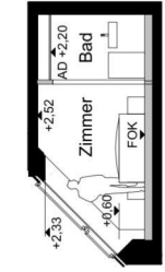
Querschnitt 1 M:1:150
