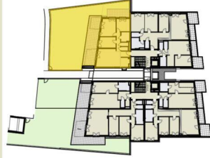
1. Dachgeschoss
