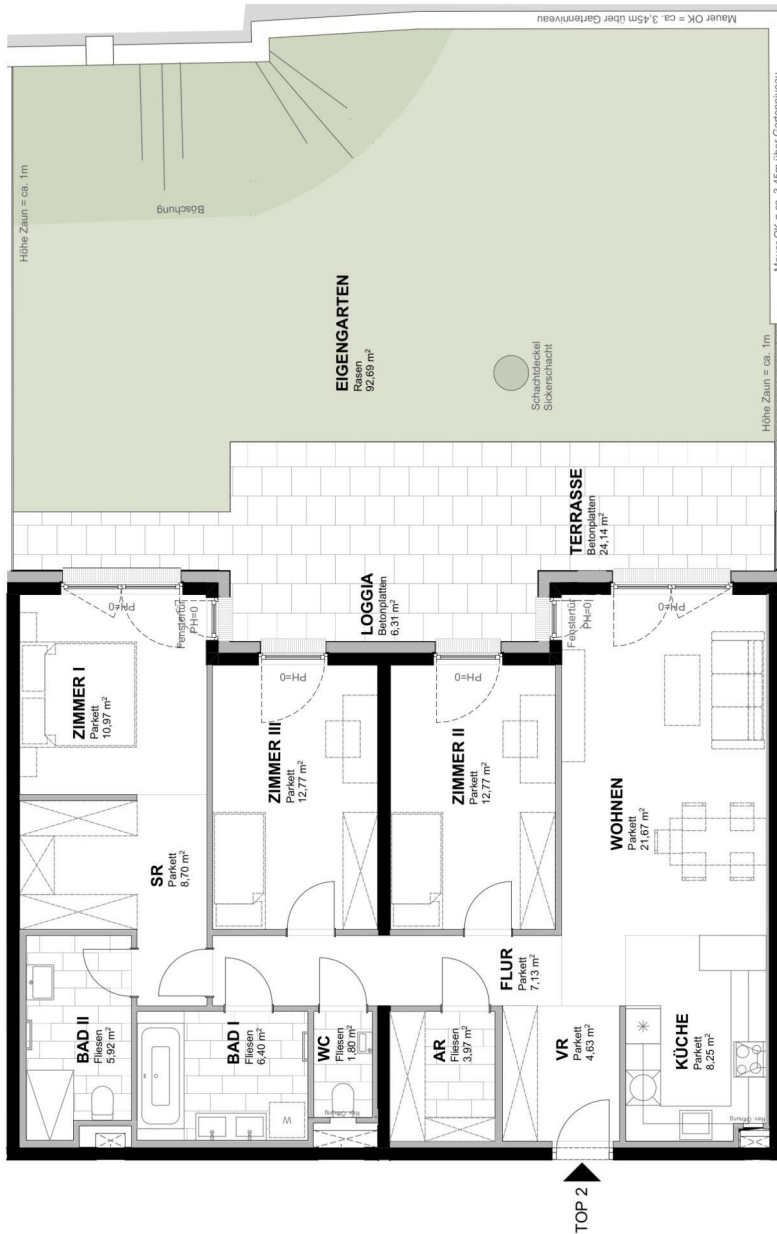
Übersichtsplan Erdgeschoss
