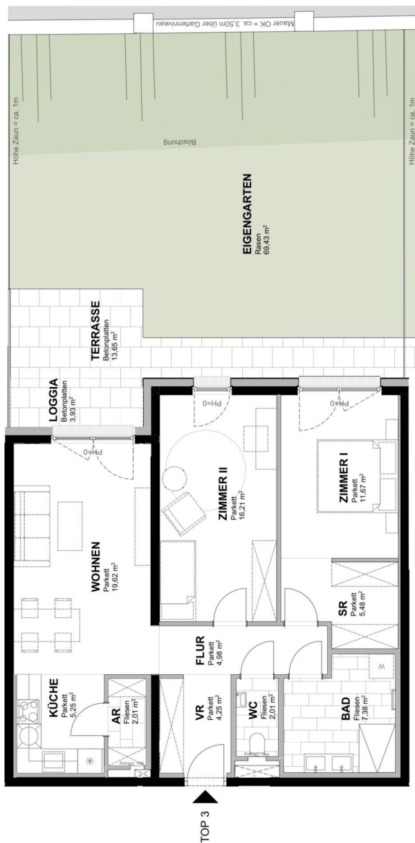
Übersichtsplan Erdgeschoss
