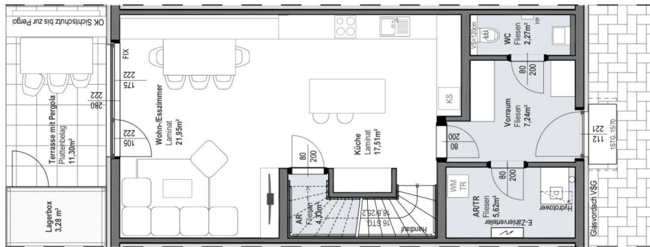
ERDGESCHOSS
