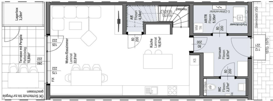
ERDGESCHOSS
