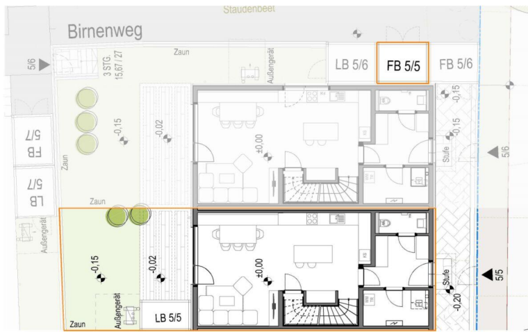
ERDGESCHOSS
