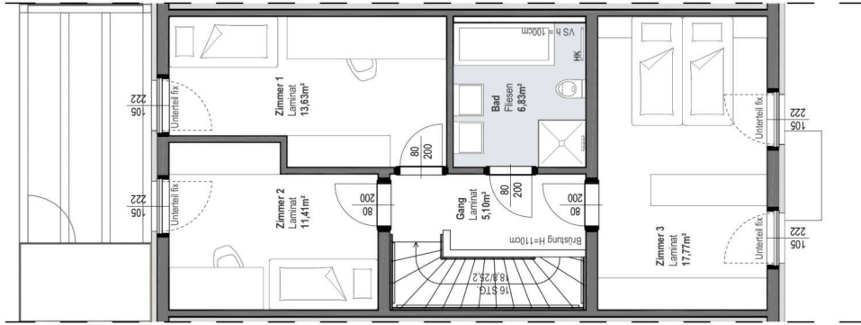
OBERGESCHOSS
